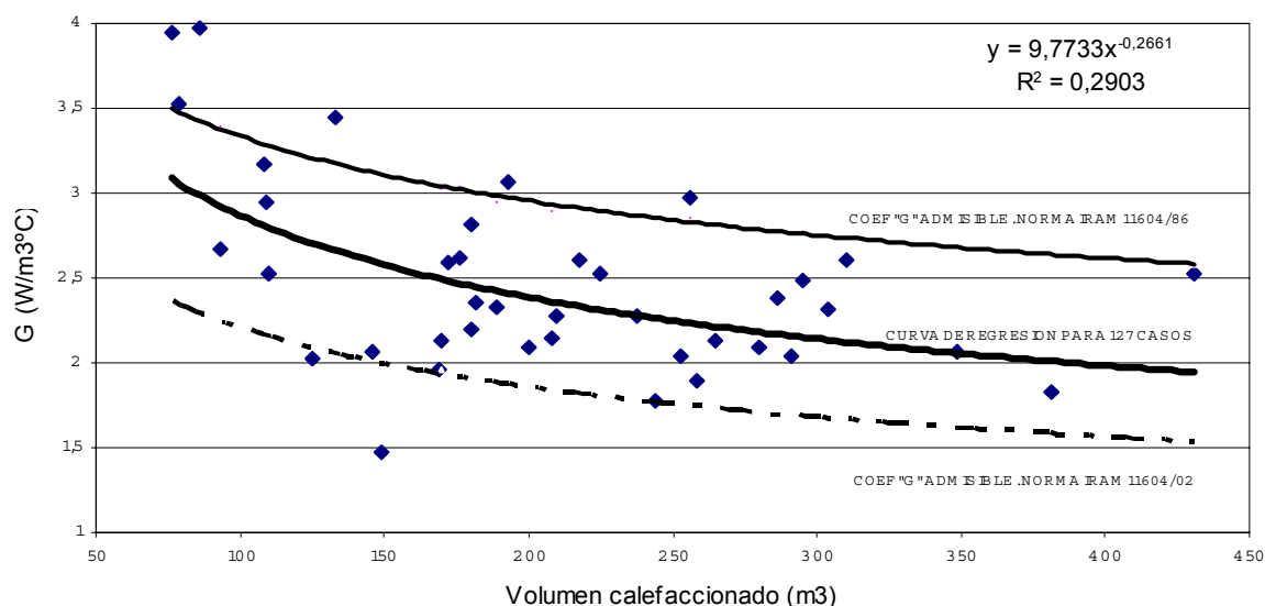
Figura 4: Comparación entre las características térmicas de la muestra y versiones de la norma IRAM 11604.
