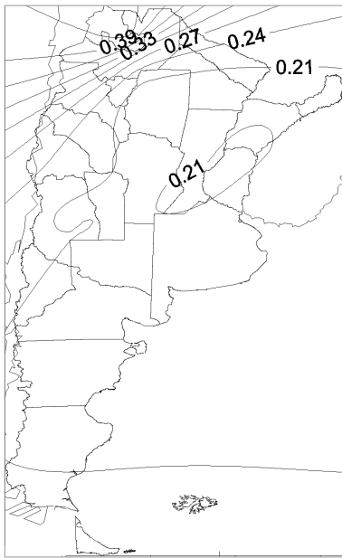
Figuras 3 y 4. Ordenada al origen (izquierda) y pendiente (derecha) para todo el país obtenidas aplicando kriging para el mes de Julio.
