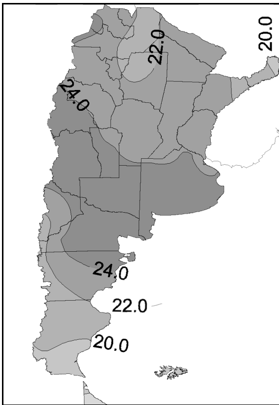
Figuras 5 y 6. Valores de energía media mensual en \text{MJ/m}^2 calculados empleando la ecuación de Ångström-Prescott para los meses de Enero (izquierda) y Julio (derecha).
