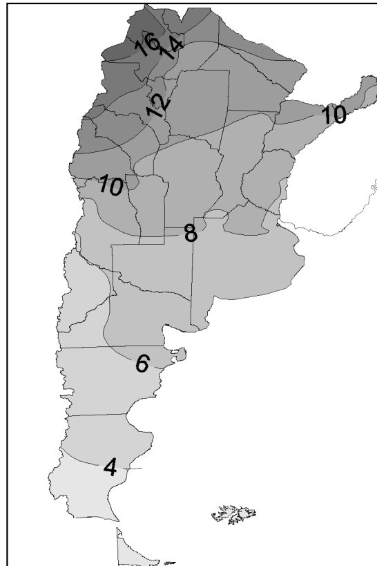
Figuras 5 y 6. Valores de energía media mensual en \text{MJ/m}^2 calculados empleando la ecuación de Ångström-Prescott para los meses de Enero (izquierda) y Julio (derecha).
