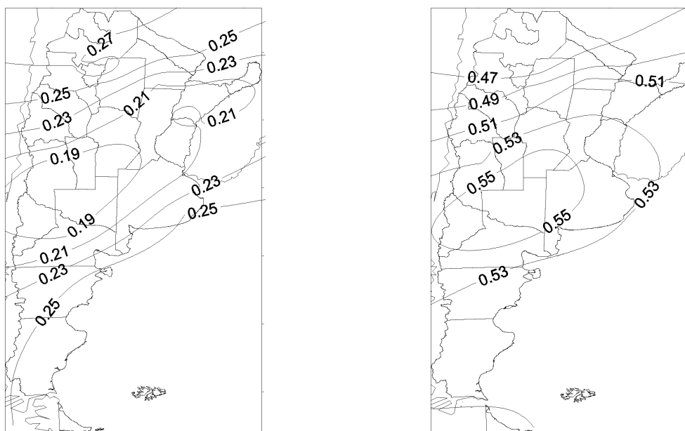
Figura 1 y 2. Ordenada al origen (izquierda) y pendiente (derecha) para todo el país obtenidas aplicando kriging para el mes de Enero.
