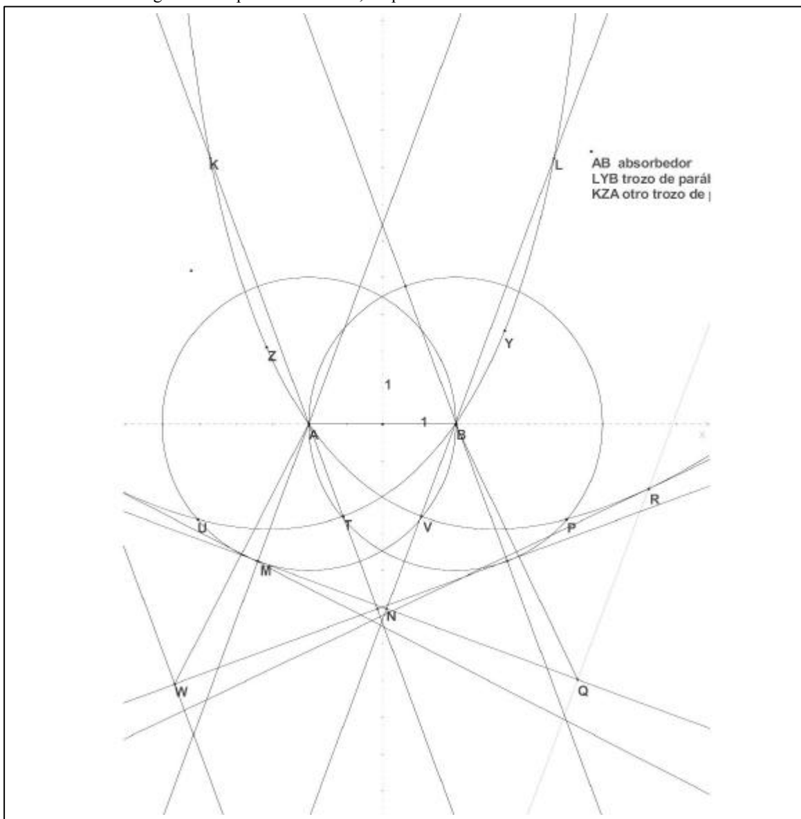
Fig. 1.- Muestra el dibujo en el Cabri con el que se obtiene el diseño del CPC compuesto por una superficie horizontal AB y los trozos de parábola AK y BL.
