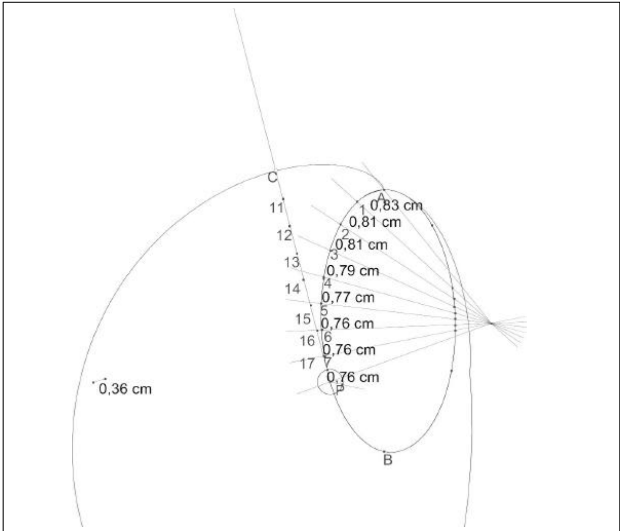
Fig. 2.- Ilustra el trazado de la involuta de la elipse AB. Se traza un punto de la involuta, el C, partiendo de un punto P y su tangente. La involuta comienza en A y en el trozo de elipse AP se marcan puntos a distancias aproximadamente iguales mediante el haz de rectas. Las distancias P-7, 7-6, 6-5, etc se transportan sobre la tangente PC para determinar el punto C. Moviendo el punto P mediante el comando "lugar" se traza la involuta cómo el conjunto de las posiciones de C al moverse P.
