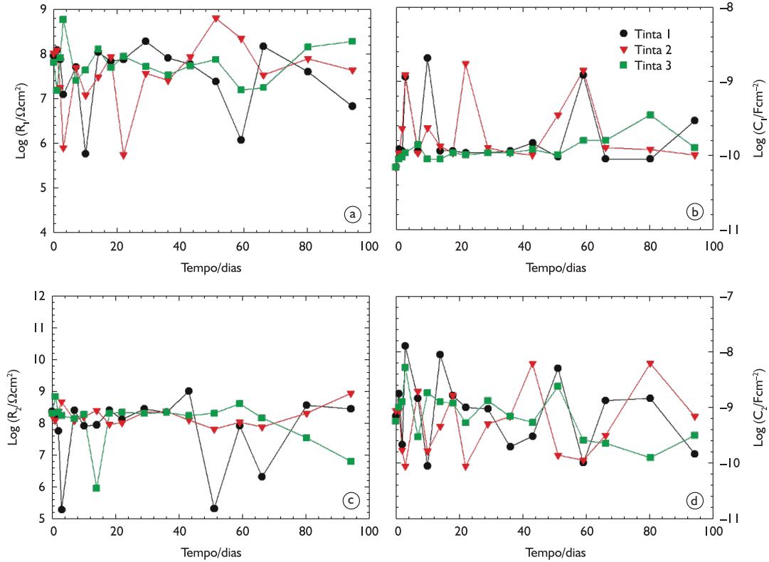
Figura 5. Evolução dos parâmetros: (a) \log R_p , (b) \log C_i , (c) \log R_2 e (d) \log C_2 , para o sistema Zn – Cr VI – revestimento orgânico pintados com três tintas, após imersão em solução 0,05 mol/L de \text{NaCl} .
