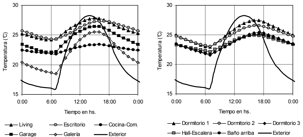
Figura 4: temperaturas simuladas de los locales de ambas plantas para clima de verano.
