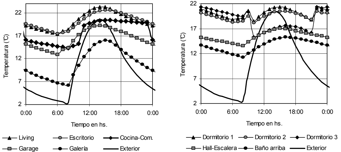
Figura 3: temperaturas simuladas de los locales de ambas plantas con calefacción auxiliar.
