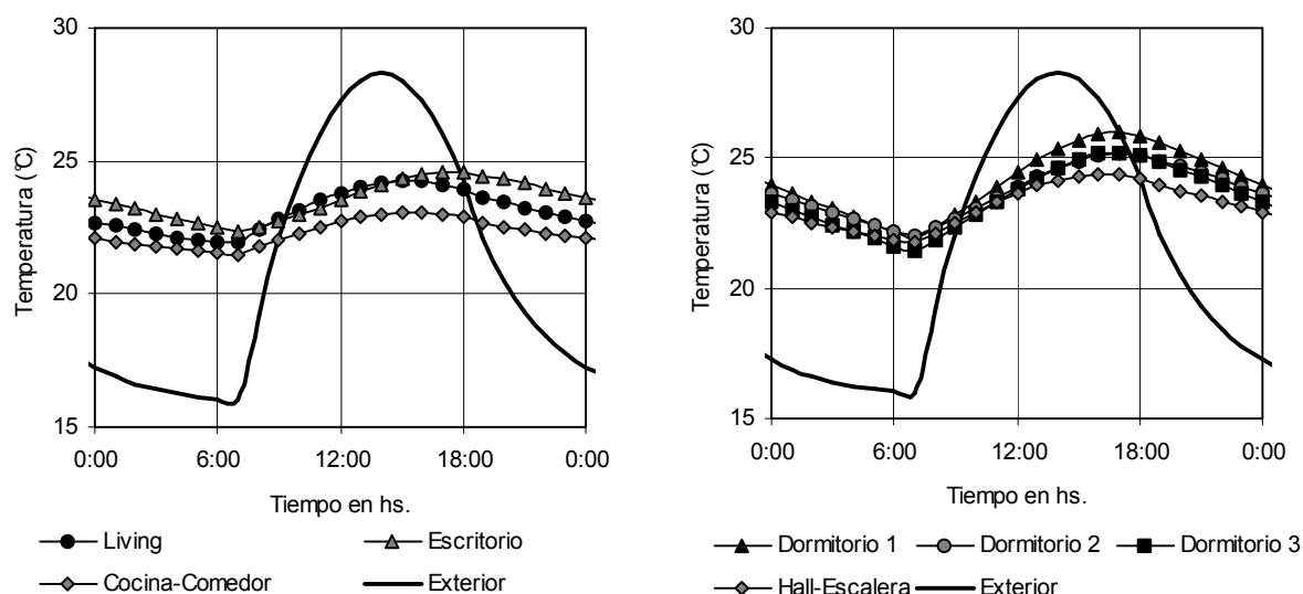
Figura 5: temperaturas simuladas de los locales de ambas plantas con ventanas apantalladas.
