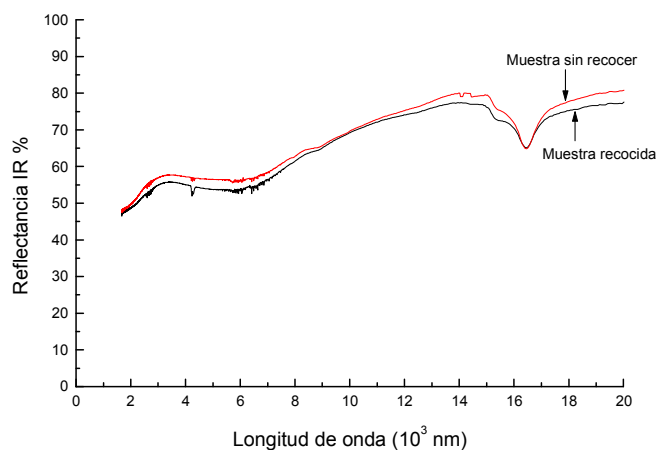
Fig.6 Espectro de reflectancia IR de un recubrimiento de Cr-Cr 2 O 3 recocido en aire a 300°C durante 30 días, comparado con su espectro de reflectancia original.
