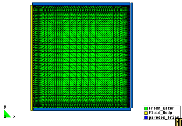
Figura 1: Dominio modelado (malla y elementos)
