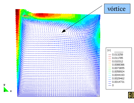
Figura 3: Campo velocidad t = t_0 + \Delta t
