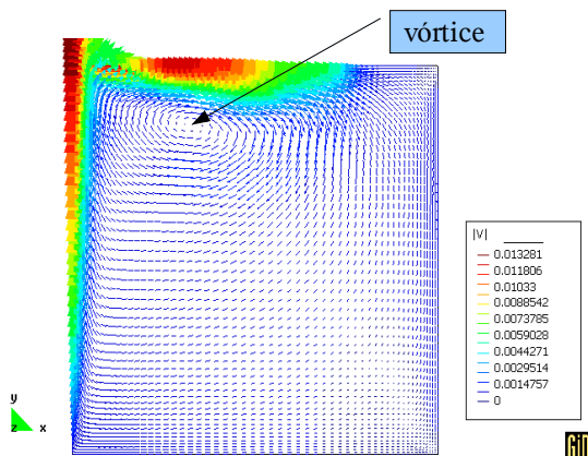
Figura 2: Campo de velocidad ( t = t_0 )
