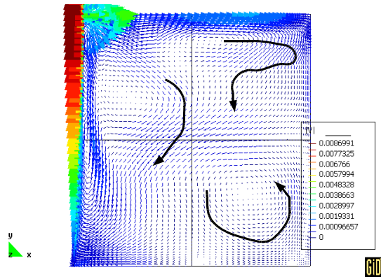
Figura 6: Campo velocidad ( t = t_0 + 130 \Delta t )
