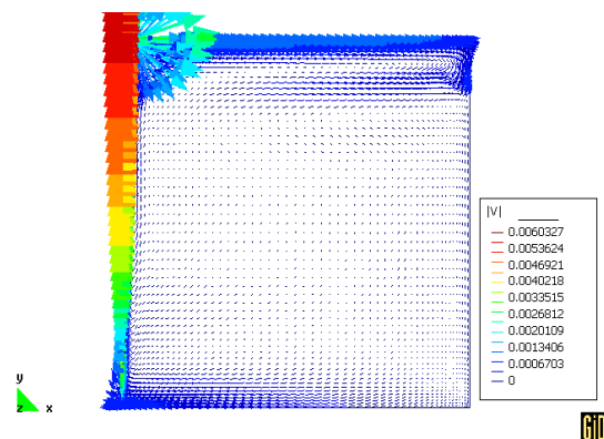
Figura 7: Campo de velocidad ( t = t_0 + 300 \Delta t )
