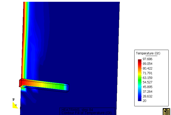
Figura 17: Temperatura sobre la aleta
