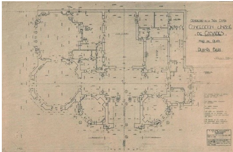
Fig. 2 Residencias de verano. Villa Concepción. Calles Bolívar y Olavaria. 1907. Arq. Faure Dujarric. Mar del Plata. Buenos Aires. Vista y planta. Fuente Municipalidad de Mar del Plata.
