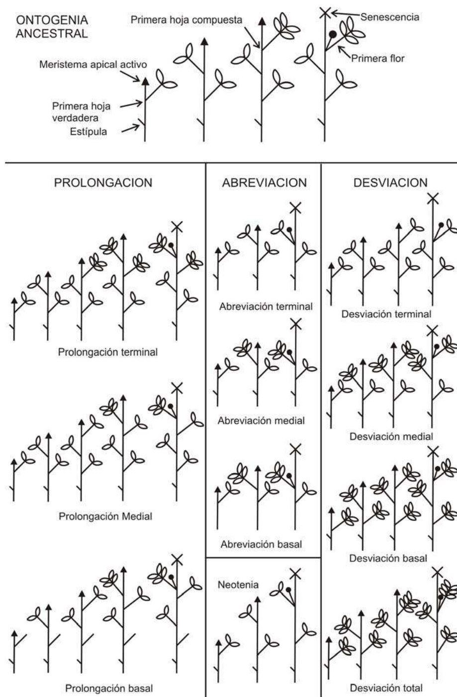
Fig. 2. Interpretación de los patrones de alteraciones ontogenéticas en la evolución de las plantas superiores de Takhtajan (1972), usando como modelo la trayectoria ontogenética de Pisum sativum tomada de Wiltshire et al. (1994). La prolongación y la abreviación pueden ocurrir en las fases finales, intermedias y tempranas del desarrollo (prolongación o abreviación terminal, prolongación o abreviación medial, y prolongación o abreviación basal, respectivamente); la desviación puede suceder en las etapas del desarrollo finales, intermedias, tempranas o todas (desviación terminal, intermedia, basal, o total, en esa orden). La neotenia es la combinación de abreviación terminal con la desviación.
