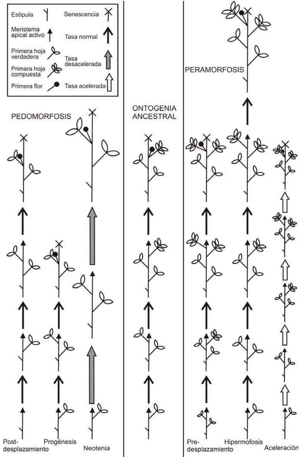
Fig. 1. Patrones y procesos heterocrónicos propuestos por Alberch et al. (1979), usando como modelo la trayectoria ontogenética de Pisum sativum tomada de Wiltshire et al. (1994).
