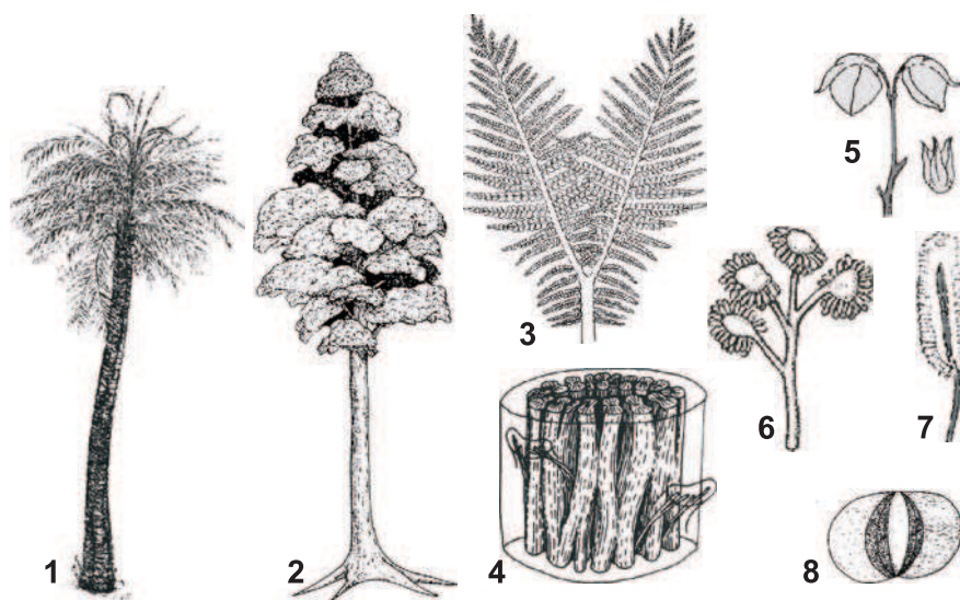
Fig. 4. Hábito y órganos de las corystospermas. 1. Reconstrucción efectuada por Petriella (1978). 2. Reconstrucción efectuada por Meyer-Berthaud et al. (1992, 1993). 3. Hoja típica de Zuberia . 4. Sección de un tronco de Rhexoxylon . 5. Esquema del órgano ovulífero correspondiente a Umkomasia . 6. Dibujo del órgano polínico perteneciente a Pteruchus . 7. Detalle de un microsporofilo. 8. Grano de polen asignable a Alisporites (Modificado de Petriella, 1978; Retallack & Dilcher, 1988; Stewart & Rothwell, 1993; Zamuner et al. , 2001; Taylor et al. 2006).
