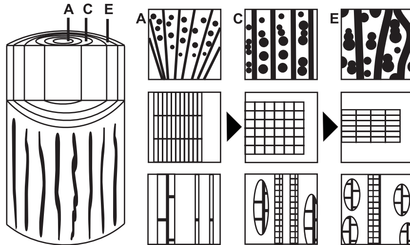
Fig. 5. Ejemplo del leño de una dicotiledónea como registro del desarrollo. A la izquierda, una sección esquemática de un tronco que abarca el xilema secundario desde la médula a la corteza. Las letras corresponden a las edades expresadas en número de estaciones de crecimiento (A, primera estación de crecimiento; C, tercera estación de crecimiento; E, quinta estación de crecimiento). A la derecha, diagramas de los cortes transversales, radiales y tangenciales, correspondientes a cada una de estas edades, mostrando los cambios ontogenéticos. En corte transversal (arriba, a la derecha), el agrupamiento de los vasos aumenta con la edad, puesto que se incrementa el diámetro de los vasos y la amplitud de los radios. En corte radial (medio, a la derecha) las células de los radios cambian de erectas a horizontales. En corte tangencial (abajo, a la derecha), las punteaduras intervasculares cambian de escalariformes a alternas poligonales, mientras que los radios llegan a ser mucho más cortos. Redibujado de Olson (2007).
