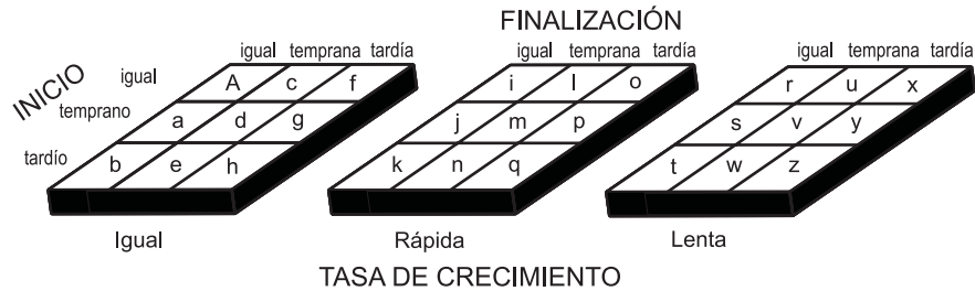
Fig. 3. Modelo de los procesos heterocronicos de Niklas (1994), en los que las tres variables ontogenéticas (inicio, finalización y tasa de crecimiento) con sus tres estados (igual, temprano/rápido y tardío/lento) son considerados como una matriz 3 x 3 x 3.
