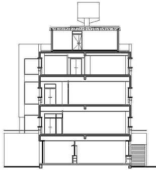
CORTE LONGITUDINAL
