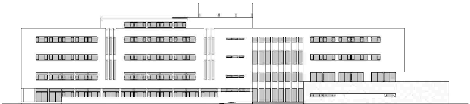
VISTAS LONGITUDINALES
