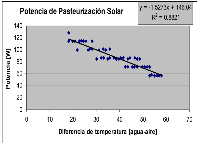
Figura 7: Potencia de pasteurización en función de la diferencia de la temperatura líquido-aire.
