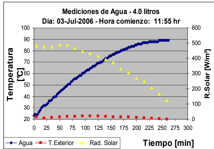
Figura 5: valores de las variables, temperatura del agua, aire y radiación solar durante el proceso de pasteurización
