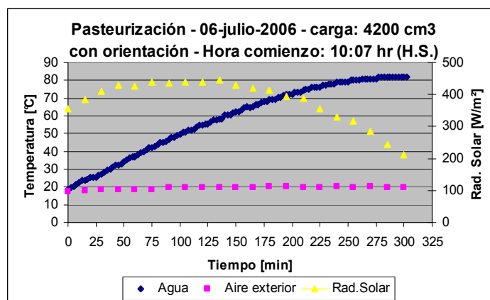
Figura 6: valores de temperatura del agua y aire y radiación solar durante el proceso de pasteurización sin precalentamiento previo.
