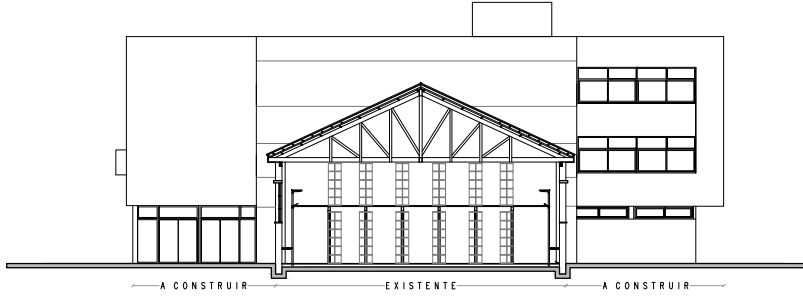
CORTE TRANSVERSAL
