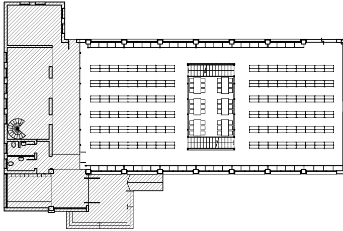
PLANTA BAJA -situación original, sectores demolidos-
