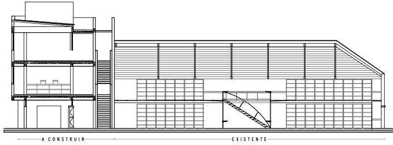
CORTE LONGITUDINAL
