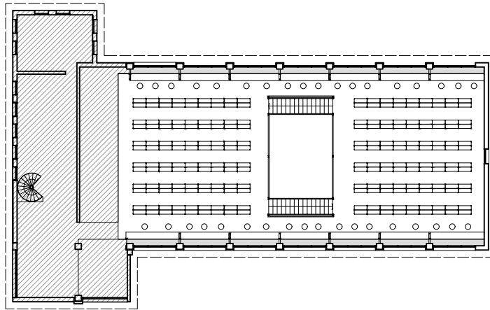
PLANTA PRIMERA -situación original, sectores demolidos-
