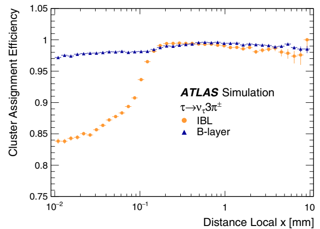
(d) \tau \rightarrow \nu_\tau 3\pi^\pm sample
