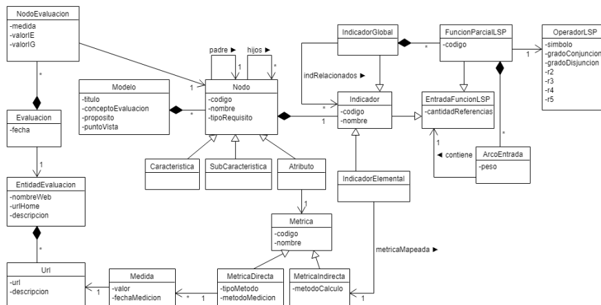
Fig. 2. Modelo de clases del dominio de M&ECalidadWeb
