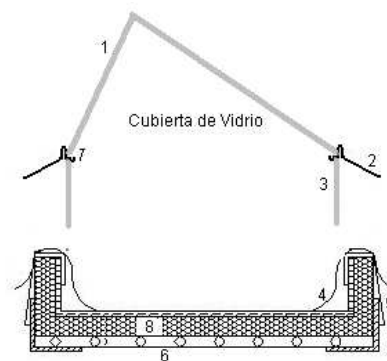
Figura 2: Corte del destilador solar de batea liviana: 1 cubierta de vidrio – 2 Perfiles de chapa acero inoxidable que sostiene la cubierta de vidrio. 3 – soportes de vidrio que apoyan sobre el fondo de la batea cerrando el receptáculo. 4 Polietileno negro. 5 Marco de hierro ángulo. 6 malla de acero de construcción. – 7 canales de agua destilada. 8 aislante térmico (Poliestireno expandido mas cartón corrugado) – 9 perfiles de chapa galvanizada que cierran la batea.
