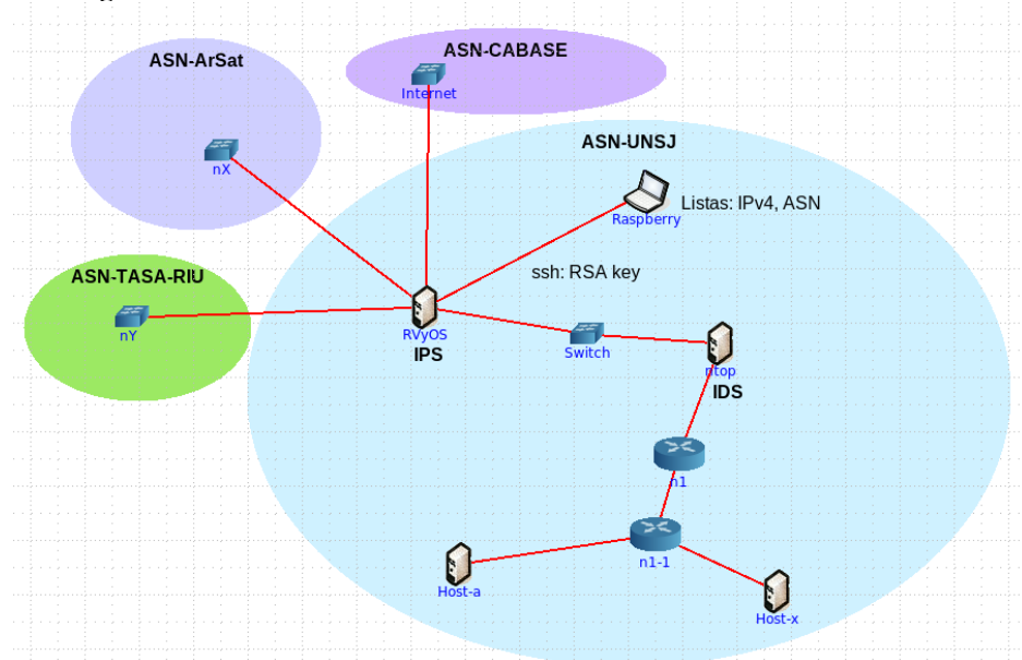
Fig. 1. Doble protección de la red: Sistema de Prevención de Intrusión IPS , donde el Router VyOS es el encargado de enviar el tráfico filtrado a la red interna de la Universidad, y el Sistema de Detección de Intrusión IDS , implementado aguas debajo de la red, complementa el filtrado del tráfico.
