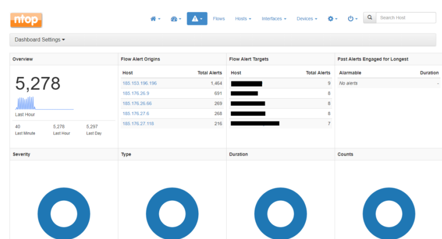
Fig 2. a) Descripción de los 5278 intentos de intrusión a la red al suspender como prueba la regla del firewall.
