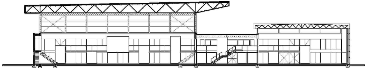
CORTE TRANSVERSAL
