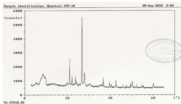
Figura 2. Difractograma .
