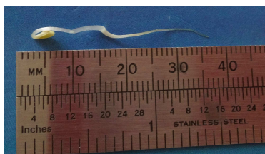
Figura 1. Medición del crecimiento en semillas de lechuga expuestas a distintas concentraciones de flavanona.
