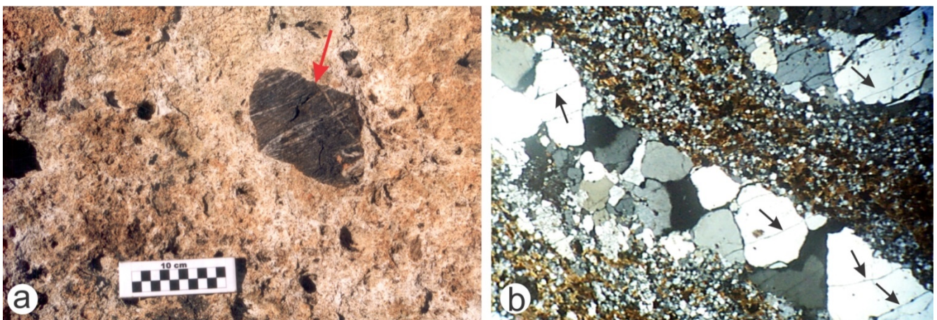
Figura 3. a. Fragmento subanguloso de esquisto cuarzo-biotítico (flecha) en facies de ignimbrita proximal. b. Fotomicrografía de la roca esquistosa donde se observan bandas de cuarzo de grano grueso alternando con bandas de cuarzo-biotita. El cuarzo grueso presenta frecuentes fracturas (flechas) oblicuas a las bandas (con analizador, ancho de la foto 7,2mm).
