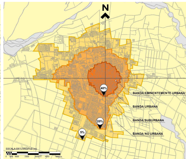
Fig 6: Bandas Urbanas Características Restituídas - 2006
