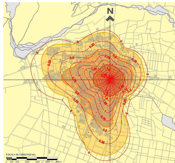
Fig. 8: Isólinas de Isla de T°C c/Límite urbano-VER.
