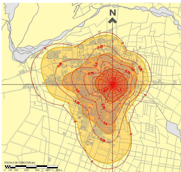
Fig. 7: Isólinas de Isla de T°C c/Límite urbano-INV.
