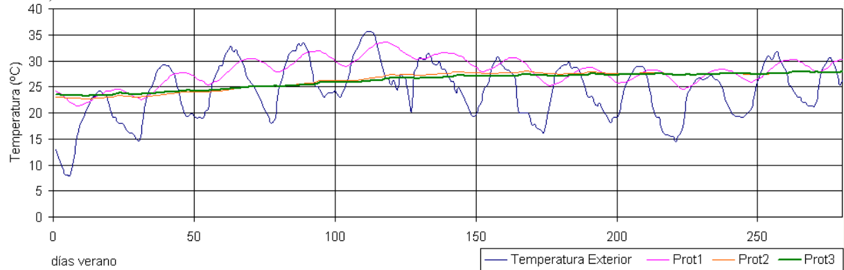
Figura 6: Comportamiento térmico veraniego de la vivienda resuelta con muros de bloques de concreto y niveles de mejora.
