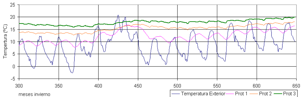
Figura 6: Comportamiento térmico invernal de la vivienda resuelta con muros de ladrillo hueco y niveles de mejora.
