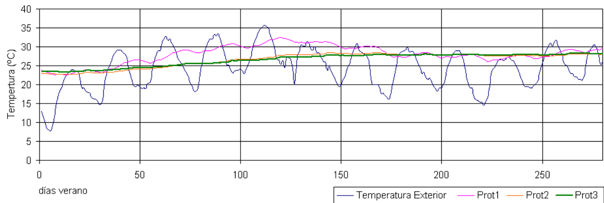
Figura 7: Comportamiento térmico veraniego de la vivienda resuelta con muros de suelo estabilizado «tapia» y niveles de mejora.
