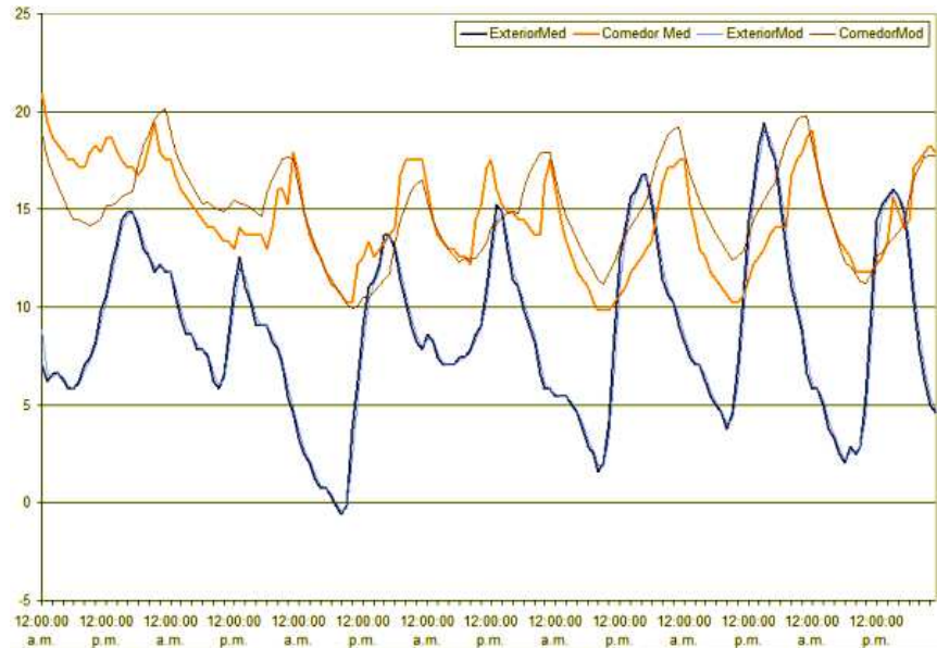
Figura 2: Validación del modelo vivienda auditada y simulado con EnergyPlus.
