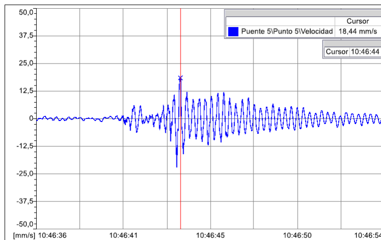
Figura 24: Amplitudes vibratorias X_N en punto 5
