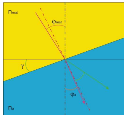
Figura 5: Ángulo \gamma de inclinación, que debe adquirir la superficie del material para que el rayo incidente \Phi_a se refracte sobre el limite de la interfaz de las superficies.
