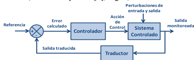
Fig. 1. Diagrama en bloques de un lazo de control a lazo cerrado.
