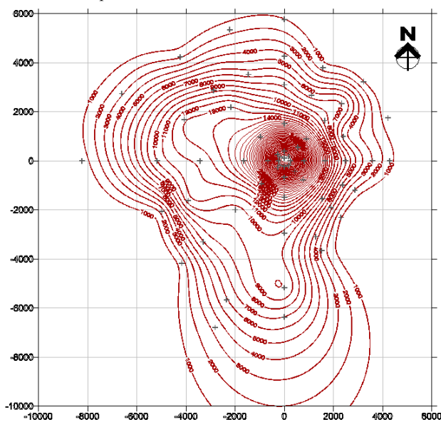
Figura 5: Isóneas representativas de DV 2008. Equidistancias de 1.000 m 3 /Ha.
