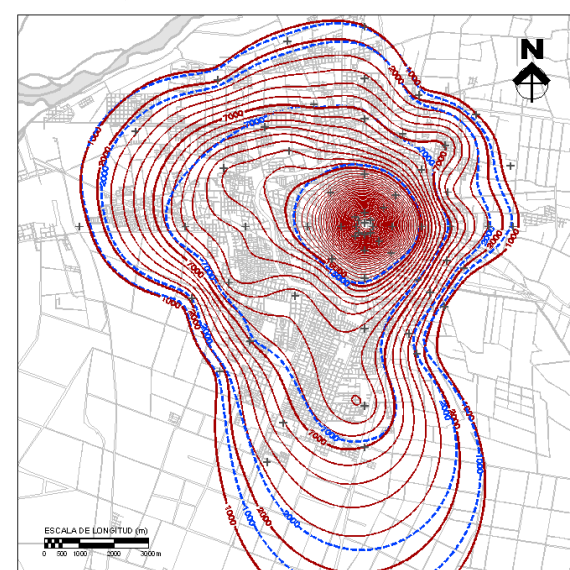
Figura 6: Distribución espacial de DV 2008 en trama urbana e Isóneas Límite de DV 2005. (15.000, 7.000 y 2.000 m 3 /Ha).
