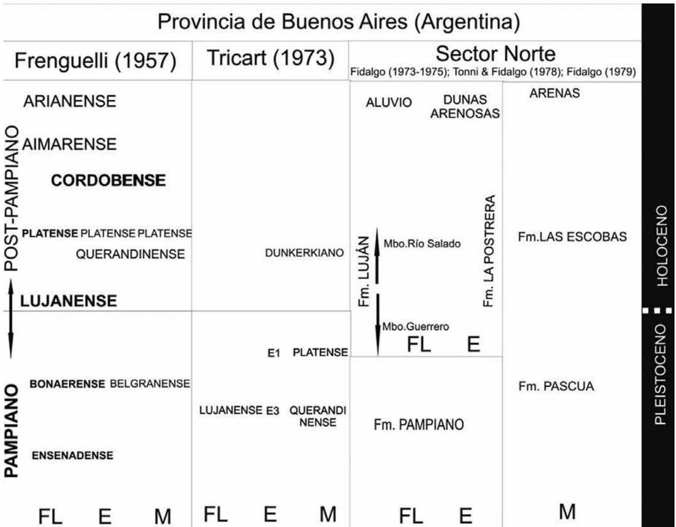
Figura 1a. Síntesis estratigráfica del Cuaternario de Argentina con énfasis en el sector bonaerense (Provincia de Buenos Aires). E: sedimentos eólicos; FL: fluviales; M: marinos. Unidades cronoestratigráficas y litoestratigráficas tradicionales para el sector bonaerense mencionadas en el texto. Fuentes de información bibliográfica en Aguirre & Whatley (1995), Tonni et al. (1999) y otras referencias allí.
