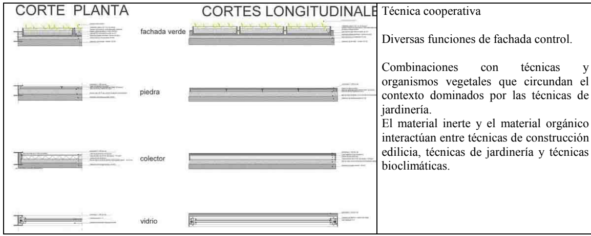
Figura 5: detalles constructivos de elementos constitutivos de la fachada multifunción.
