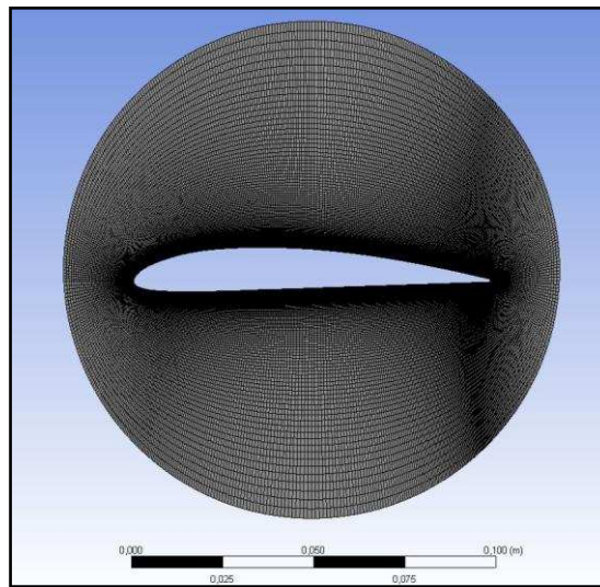
Figura 3: Detalle de la malla en el bloque correspondiente al perfil para el modelo k-\omega SST
