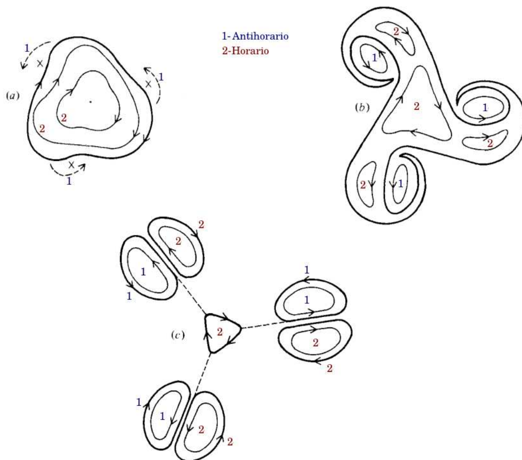
Figura 15: Diagrama esquemático del movimiento durante la formación de vórtices. En (a) las cruces marcan los puntos de acumulación de vorticidad, donde el movimiento antihorario se desarrolla. Imagen obtenida de la publicación de Griffiths y Linden (1981).
