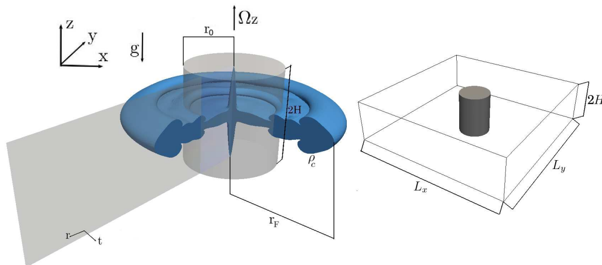
Figura 2: Esquema de configuración para las intrusiones cilíndricas. El dominio de dimensiones L_x \times L_y \times H se encuentra rotando a una velocidad angular \Omega_z alrededor del eje vertical z que pasa por el centro del dominio.
