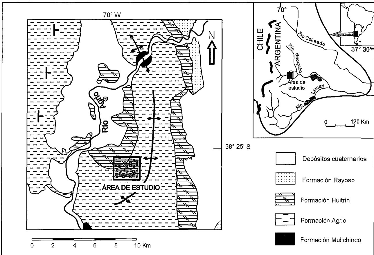
Figura 1.- Mapa de situación y esquema geológico del área de estudio.
