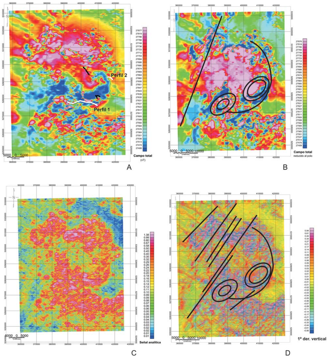
Figura 4. - Mapas magnéticos de la caldera de Piedra Parada. A: Campo magnético total y situación de los perfiles magnéticos. b: Mapa del campo magnético total reducido al polo. c: Mapa de señal analítica. d: 1ª derivada vertical del campo reducido al polo. En los mapas B y C se han indicado las estructuras magnéticas más significativas.
