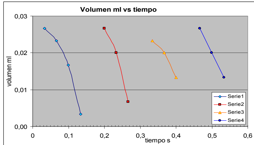
Figura 11. Volumen de agua desplazado en función del tiempo
