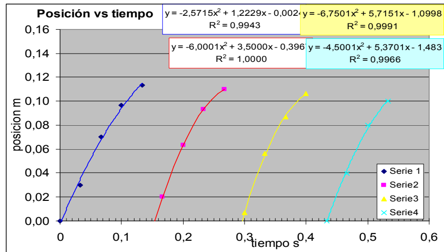
Figura 10. Posición del menisco en función del tiempo.
