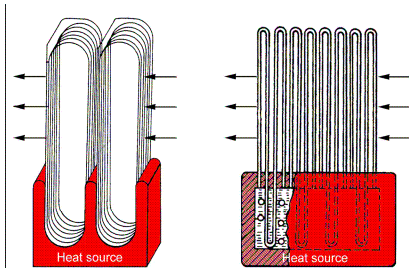
Figura 1. Heat pipes pulsantes descritos por Akachi (1993-1996).
