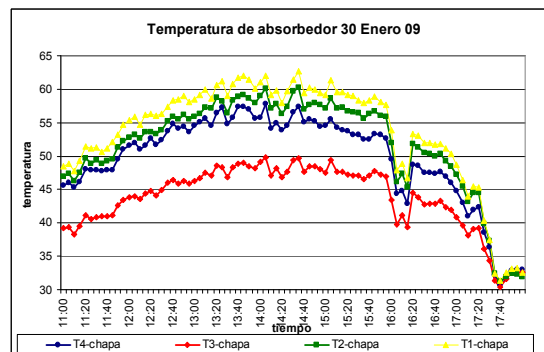
Figura 15: Distribución de temperatura, absorbedor 30/01
