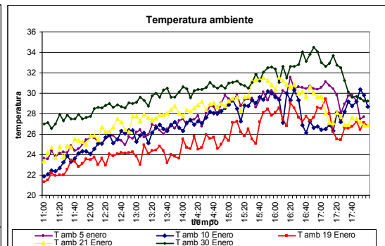
Figura 10: Distribución de temperatura ambiente.
