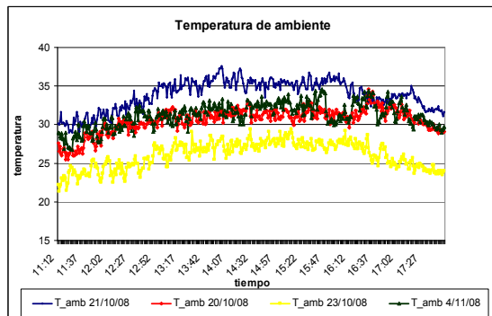
Figura 4: Distribución de temperatura ambiente
