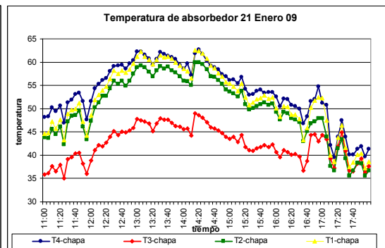
Figura 14: Distribución de temperatura, absorbedor 21/01
