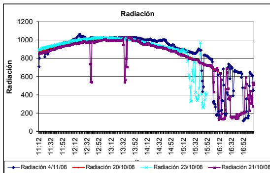
Figura 3: Distribución de radiación
