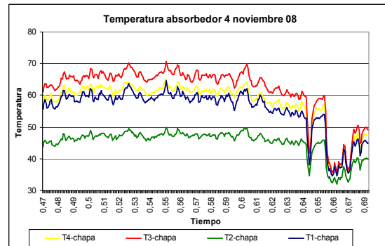
Figura 8: Distribución de temperatura, absorbedor 4/11
