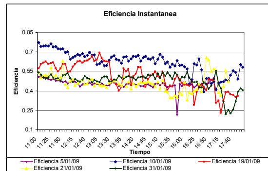
Figura 17: Eficiencia instantánea colector de matriz porosa.
