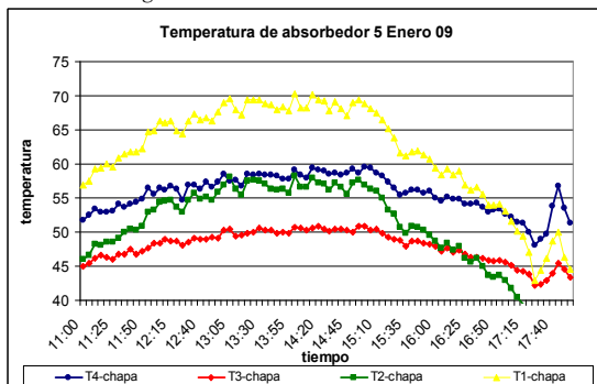
Figura 11: Distribución de temperatura, absorbedor 5/01
