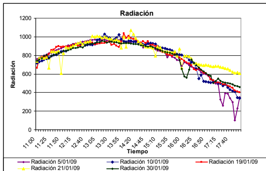
Figura 9: Distribución radiación
