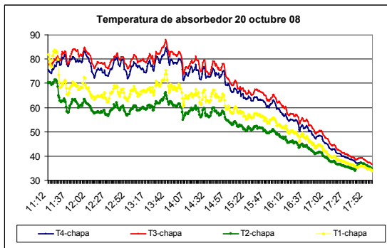
Figura 5: Distribución de temperatura, absorbedor 20/10
