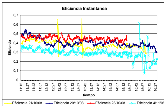
Figura 16: Eficiencia instantánea colector de chapa simple.
