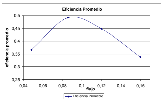
Figura 18: Eficiencia promedio colector de chapa simple.
