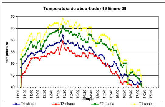
Figura 13: Distribución de temperatura, absorbedor 19/01
