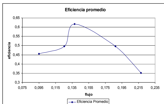
Figura 19: Eficiencia promedio colector de matriz porosa.
