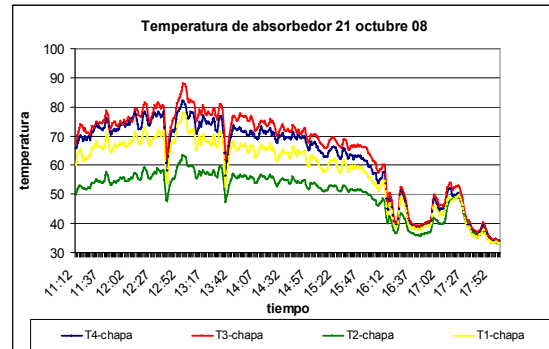
Figura 6: Distribución de temperatura, absorbedor 21/10
