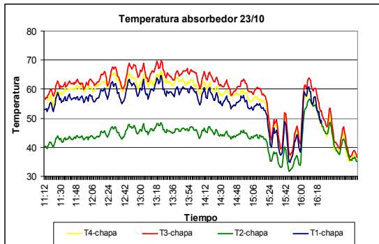
Figura 7: Distribución de temperatura, absorbedor 23/10
