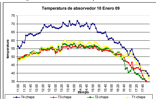
Figura 12: Distribución de temperatura, absorbedor 10/01
