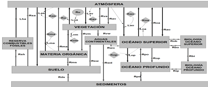
Figura 5: Modelo de reservorios para la estimación del balance de carbono.
