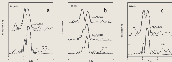
Figura 1. a) Transformadas de Fourier (FT) das EXAFS ponderadas com k^3 e suas correspondentes configurações de dispersão única para AuPd100-nNaLTA e Au foil medidas na borda Au-L3; b) Idem a) para Au50Pd50NaLTA, Pd65Pt35NaLTA e folha de Pd medida no limite Pd-K e c) idem a) para Pd65Pt35NaLTA e Pt foil medidas no limite Pt-L3. Linhas pontilhadas, dados experimentais; linhas sólidas, dados instalados. Os espectros de absorção de raios X foram recolhidos à temperatura ambiente sob 100 kPa Ar após o tratamento com H 2
