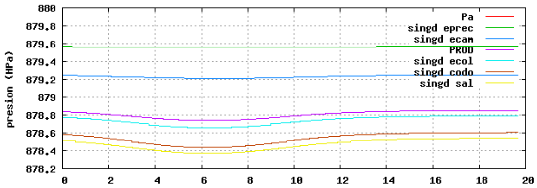
Figura 8: Perdidas de carga en el secador.
