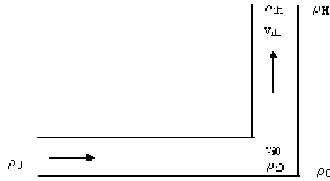
Figura 1: Esquema de la chimenea solar propuesta. Entre la cubierta y el absorbedor existe una cámara cerrada de aire.
