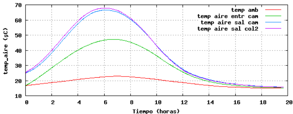
Figura 7: Resultados de la simulación. Temperatura del flujo de aire en los distintos elementos del secador.
