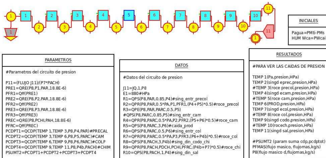
Figura 5: Circuito de flujo por caída de presión. La resistencia R5 describe la caída de presión por carga de producto.
