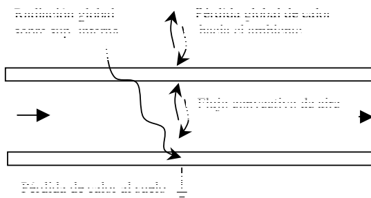
Figura 3: Esquema simplificado de las transferencias de energía en el sistema.
