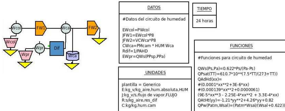
Figura 6: Circuito de flujo de masa por diferencias de humedad absoluta.
