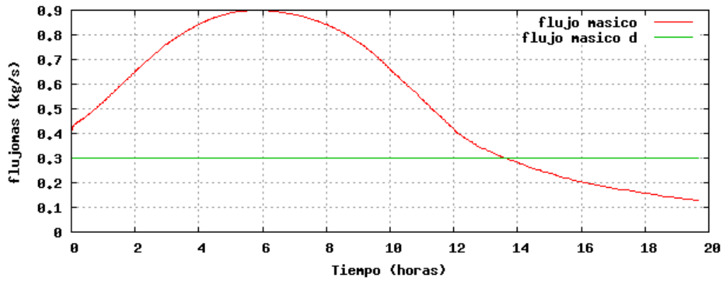
Figura 9: Flujo de aire en el interior de la cámara de secado. Flujo de diseño.
