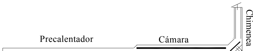
Figura 2: Esquema del secador simulado. El gráfico no tiene esta realizado a escala.
