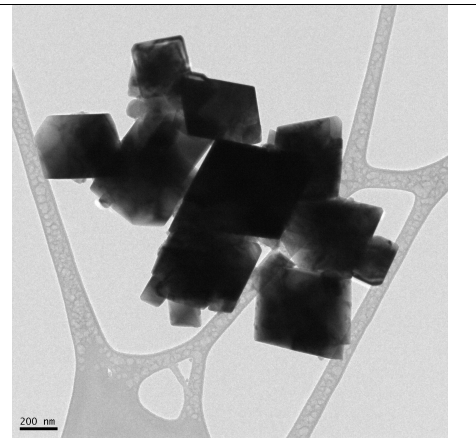
Figura 3. TEM del pigmento de \text{Co}_3\text{O}_4 sintetizado usado en la película.
