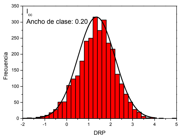
Figura 5: Histograma de las DRP(CIC CNEA, No CIC Emcore) y su curva gaussiana de I_{cc} para las 2986 celdas.
