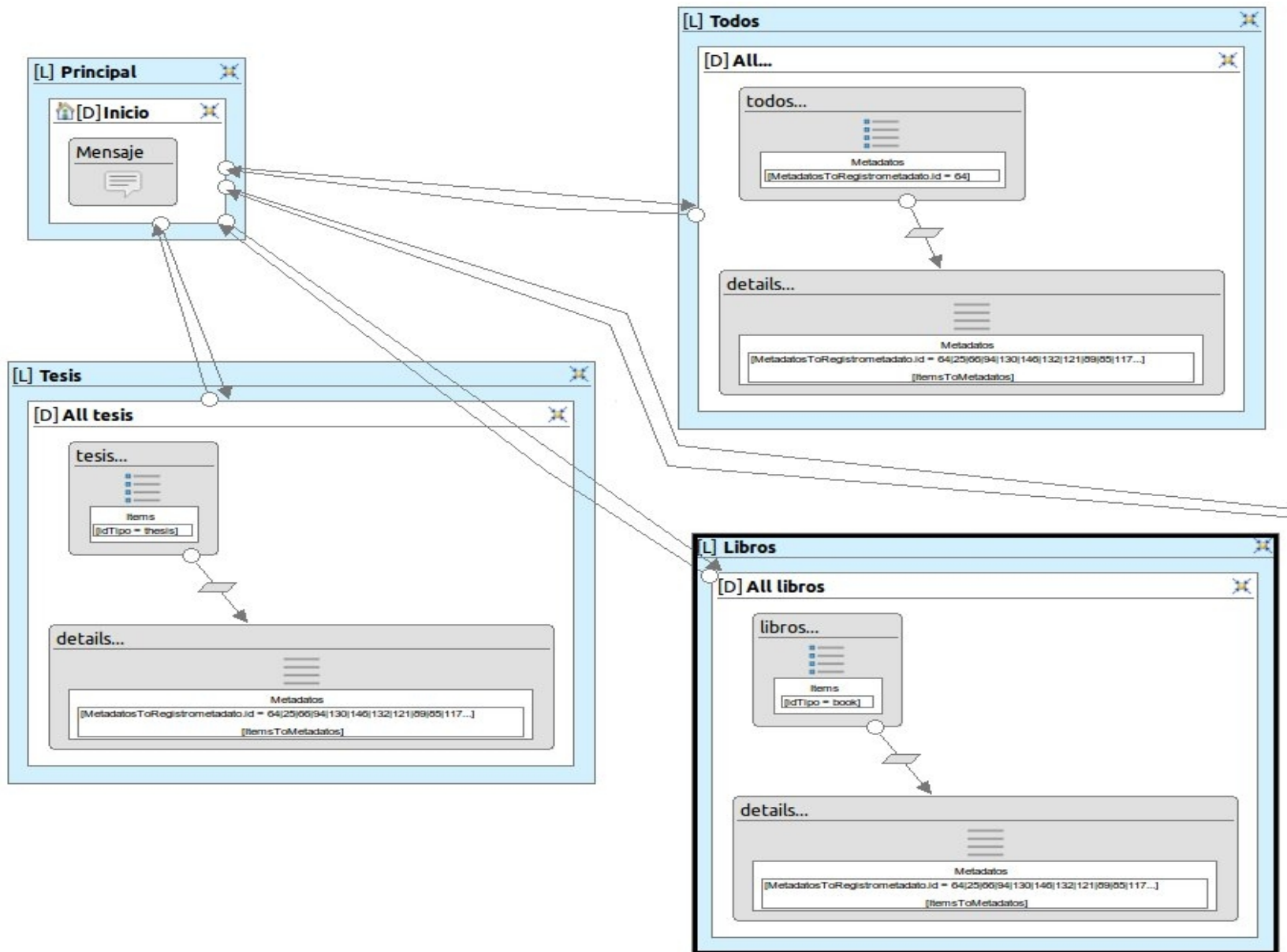
Modelo navegacional – WebRatio. Fuente: Desarrollo propio
