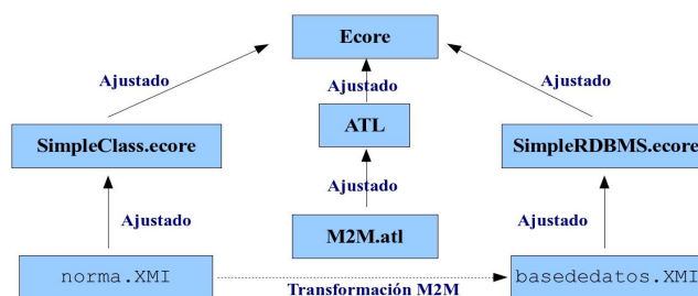
Fig. 3. Esquema de transformación M2M
