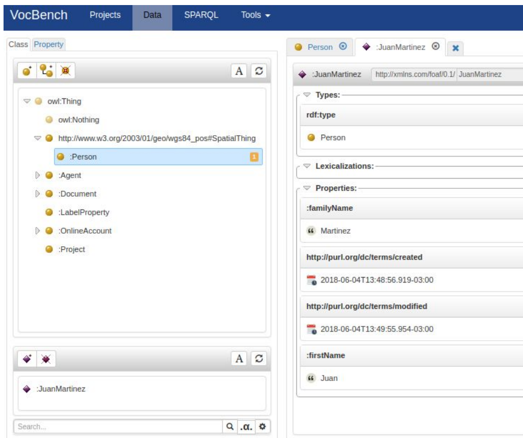
Figura 10. Creación de instancia del tipo foaf:Person
