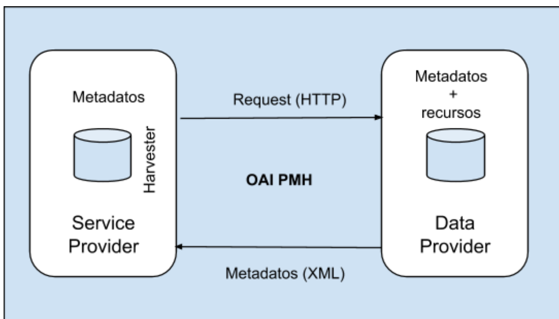
Figura 5. Protocolo OAI-PMH
