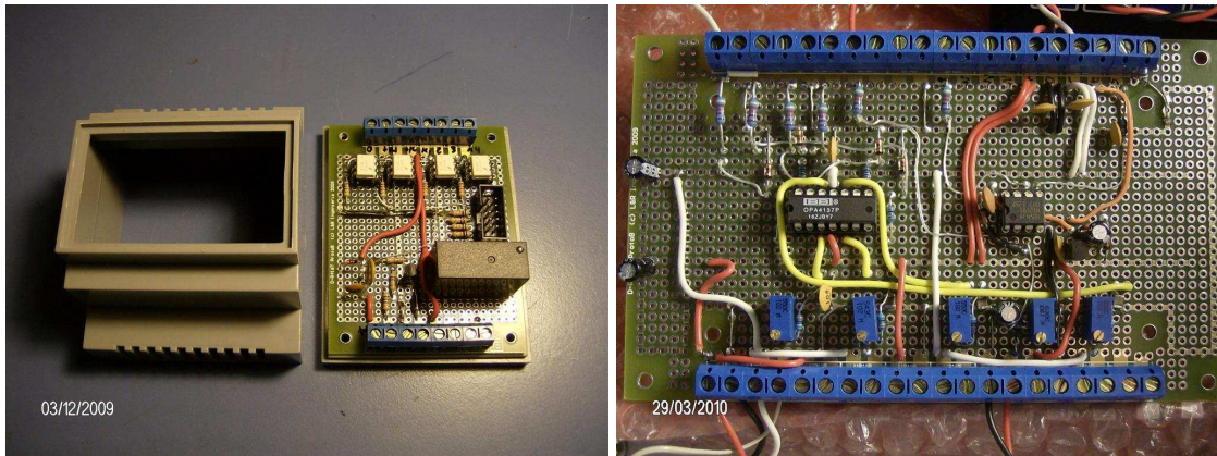
Figura 6 (izq) – Interfase lógica Diesel/Inverter (instalada y en funcionamiento desde 12/09) y (der) Entrada de Canales Analógicos (ambas placas basadas en proto-boards desarrollados por L&R Ingeniería)
