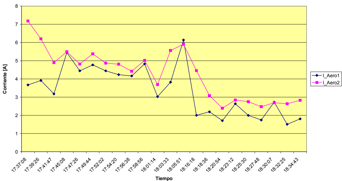
Figura 10 – Primeras mediciones con el SISMED/C descargadas del pen-drive a la Notebook 24-5-2010
