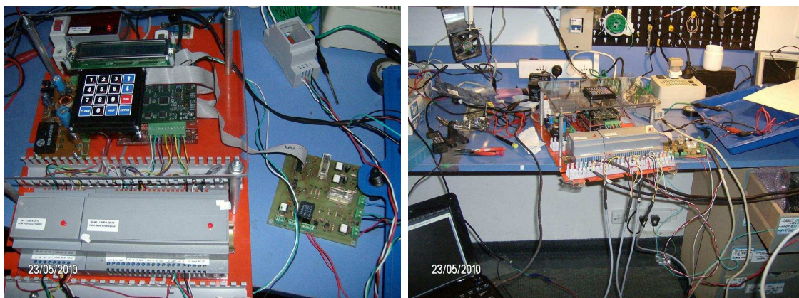
Figura 8 (izq) Armado final del equipo SISMED/C + Placa Interfase Desele (der) Calibración del SISMED/C – 23/5/2010
