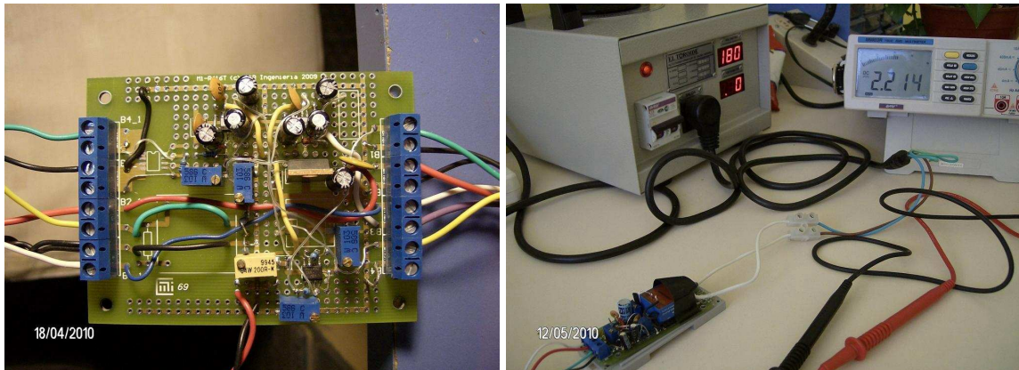
Figura 7 (izq) Placa MI/Glencross- conversión RMS a CC de señales Iac/Vac de sensores LEM a la salida del Inverter, y (der) Ensayo en laboratorio UNPA de Placa VIN-Diesel /Glencross-(medición tensión Fase/N del Diesel)
