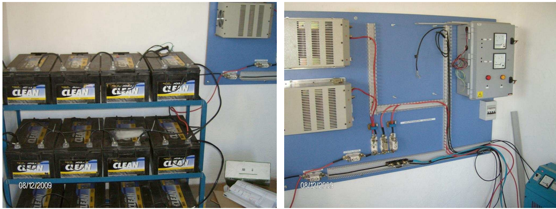
Figura 4 (izq) – Banco de Baterías en montaje y (der) tablero principal en montaje
