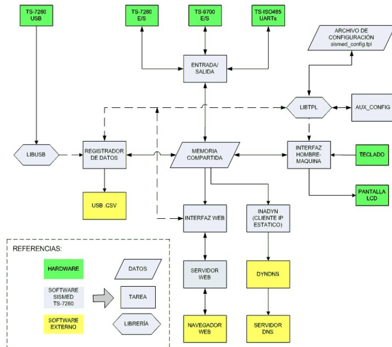
Figura 9 - Estructura del software SISMED/C
