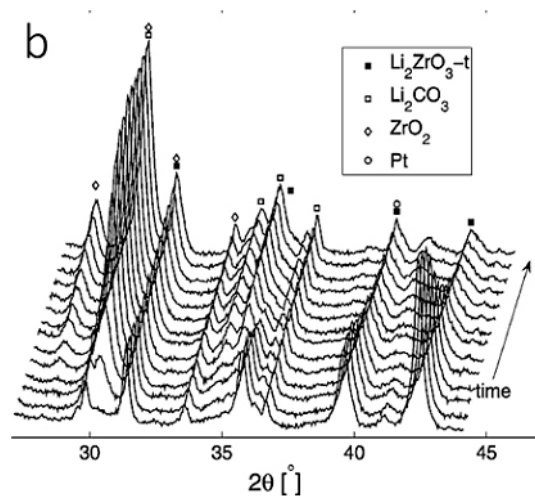
Figura 7. b. Difractogramas de \text{t-Li}_2\text{ZrO}_3 luego de múltiples ciclos de absorción-desorción de \text{CO}_2 a 575\text{ }^\circ\text{C} y 650\text{ }^\circ\text{C} , respectivamente. Imágenes obtenidas de Ochoa-Fernández et al. [64], [65]
