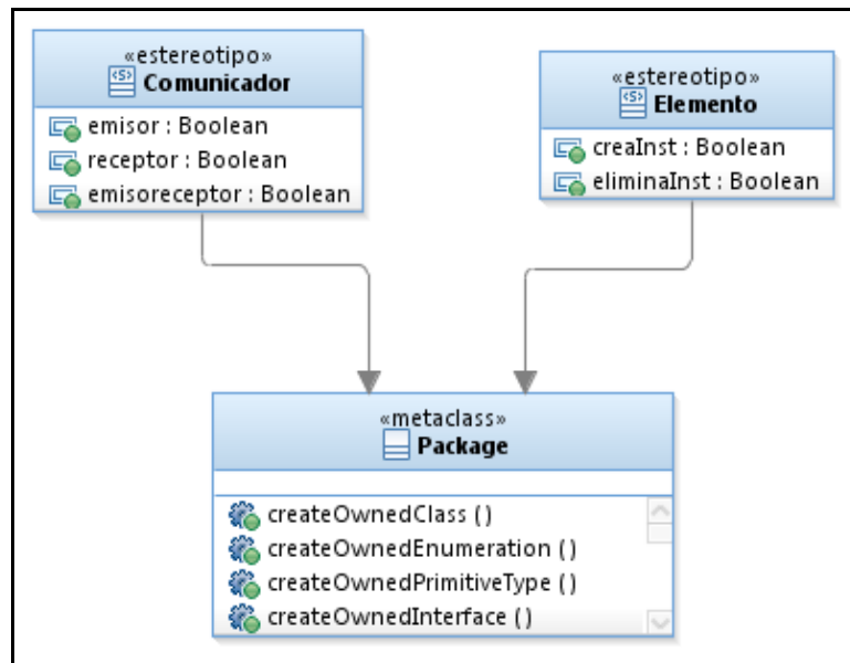
Fig. 3. Perfil de comportamiento Nivel 1
