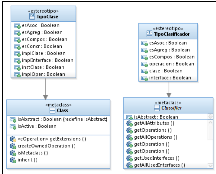
Fig. 2. Perfil DFP Nivel 0
