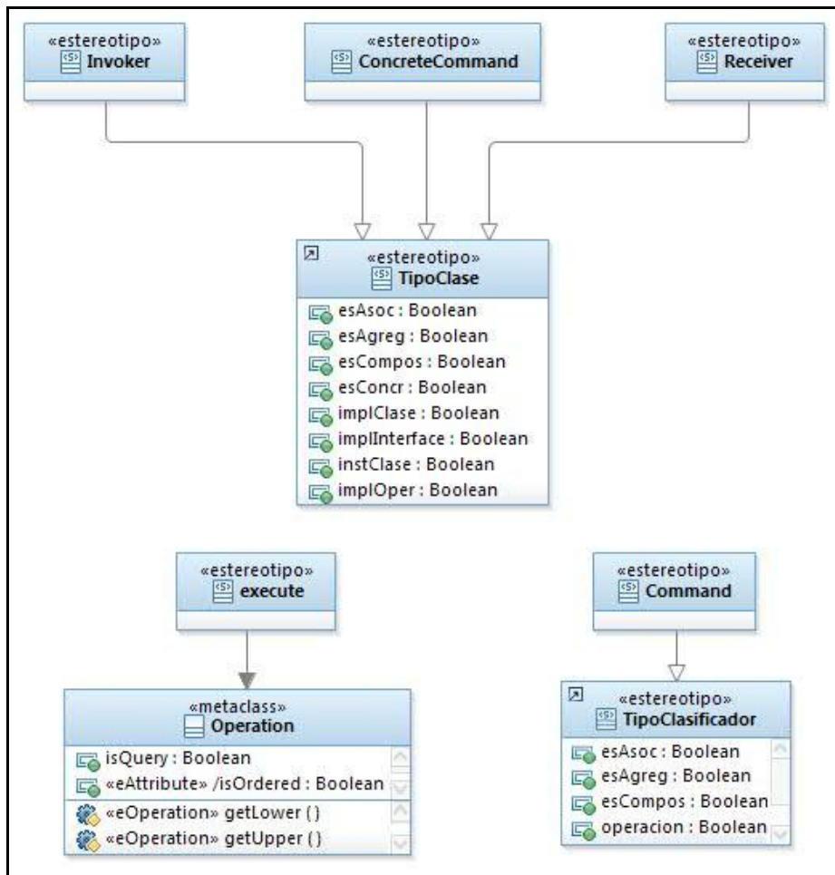
Fig. 4. Perfil del patrón Command: nivel 2
