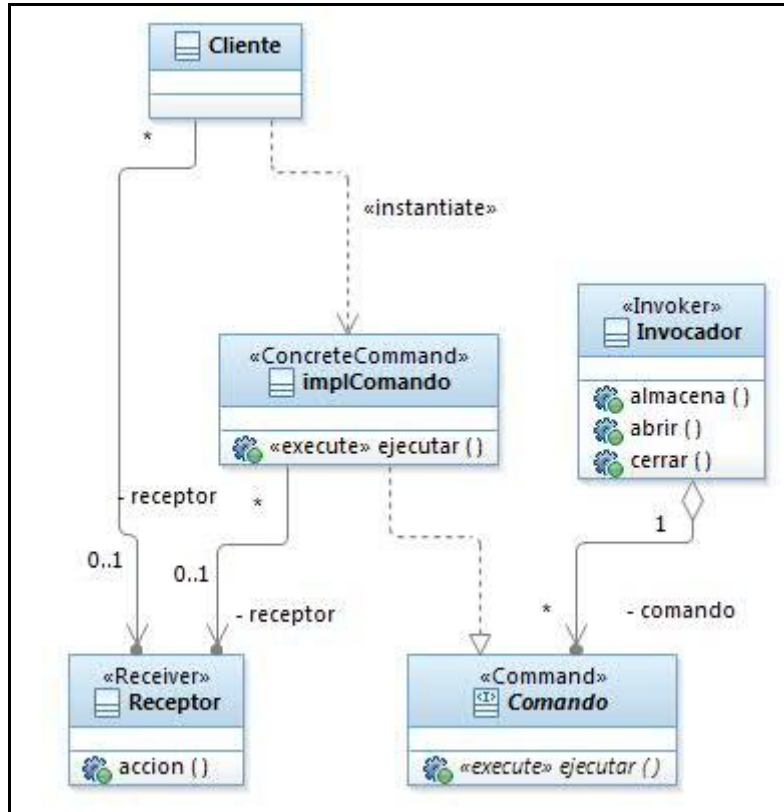
Fig. 5. Perfil Command aplicado a un diagrama de clases.
