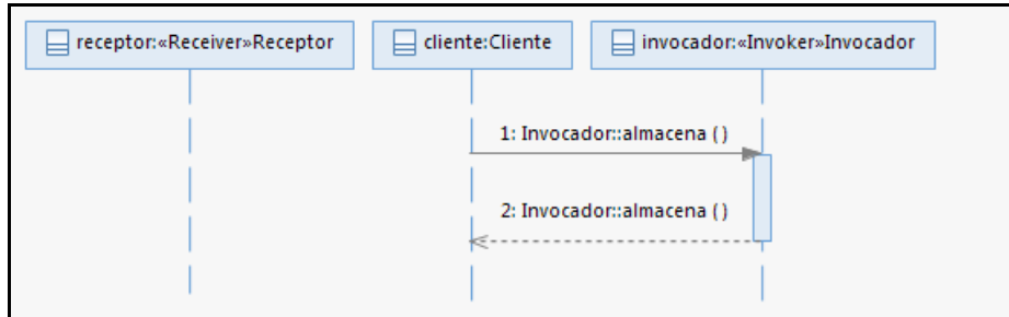
Fig. 7. Diagrama de secuencia inválido: Creación y ejecución de Command.
