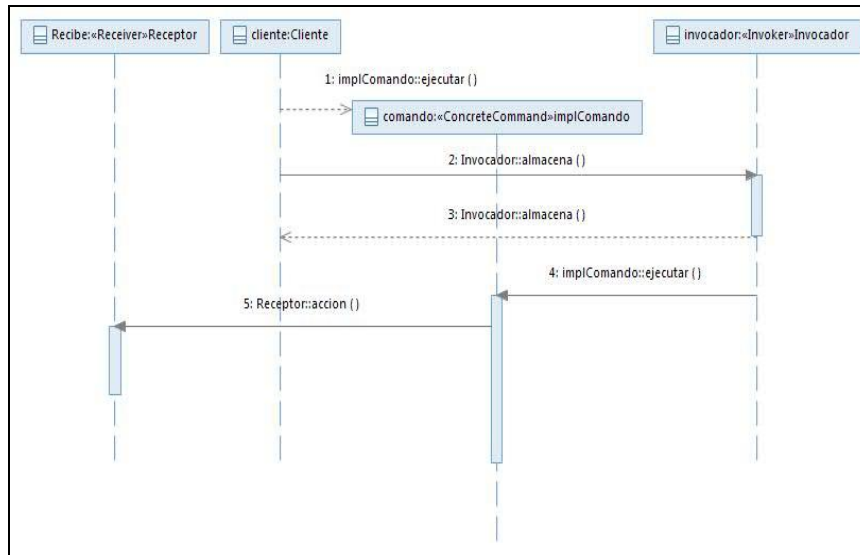
Fig. 6. Diagrama de secuencia: Creación y ejecución de Command.
