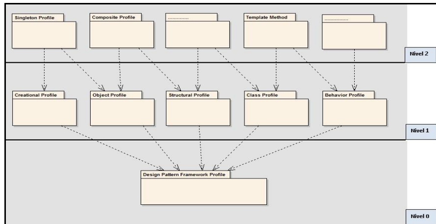
Fig. 1. Arquitectura para patrones usando perfiles UML
