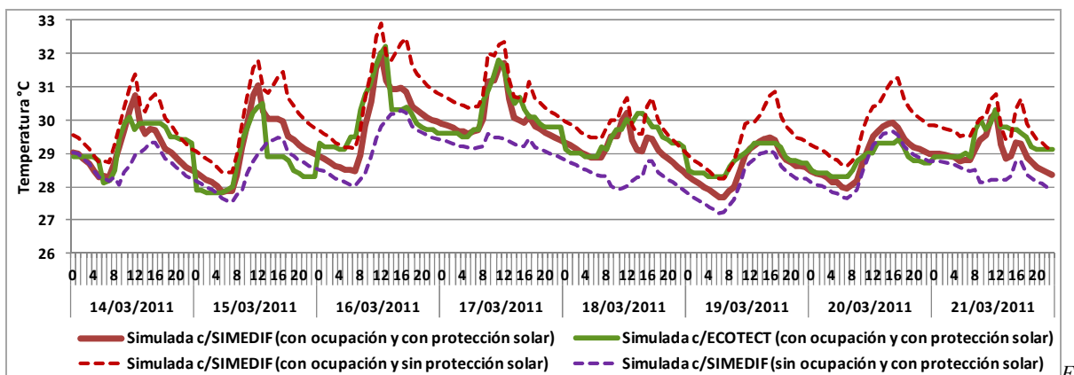
Fig. 6. Contrastación de temperaturas simuladas con SIMEDIF y ECOTECT. Aula Amarilla - ALA 1
