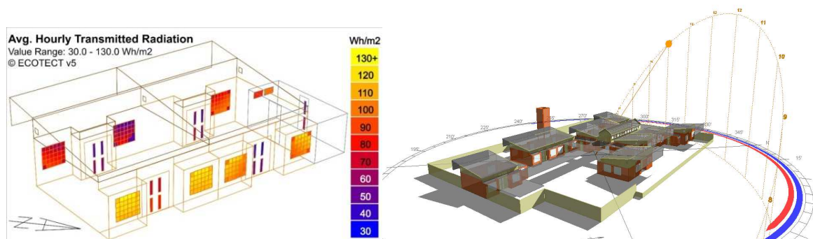
Figura 2: Izq. Gráfico de Radiación solar Incidente (Promedio) sobre áreas vidriadas del Módulo Aula Naranja. Der. Modelo renderizado con trayectoria solar, día de sol pleno, 15:00 h. Elaboración propia mediante Ecotect.
