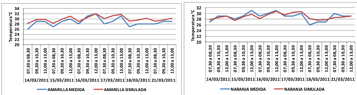
Fig. 5. Contrastación de temperaturas medidas y simuladas con SIMEDIF por rangos horarios.
