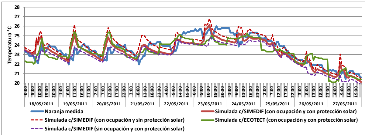
Fig. 4. Contrastación de temperaturas medidas y simuladas bajo diferentes parámetros. Aula Naranja - ALA 2
