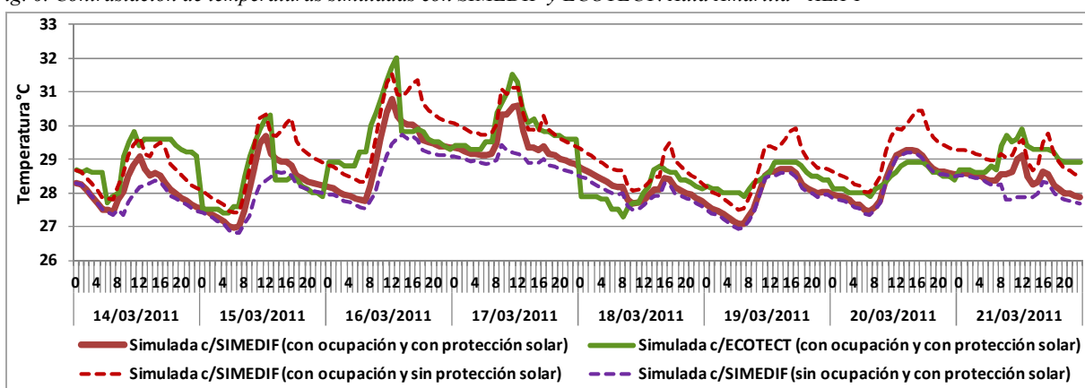
Fig. 7. Contrastación de temperaturas simuladas con SIMEDIF y ECOTECT. Aula Naranja - ALA 2
