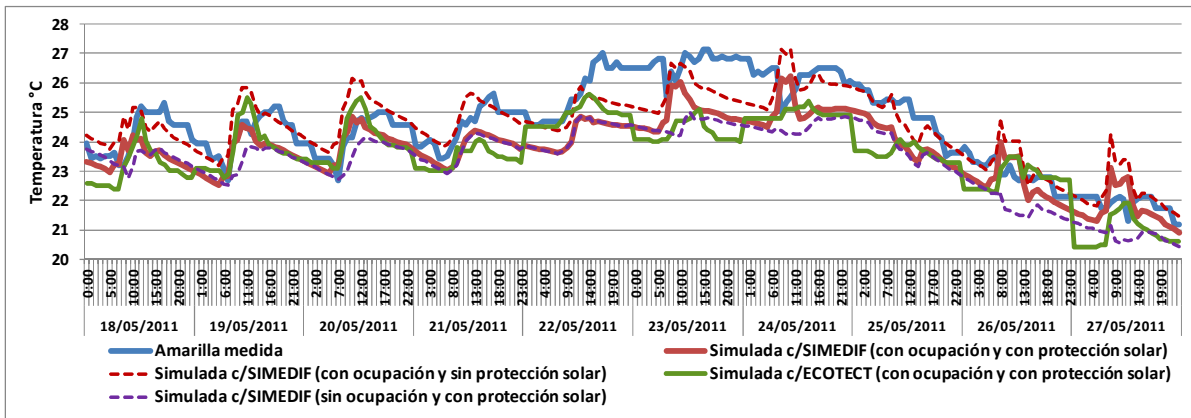
Fig. 3. Contrastación de temperaturas medidas y simuladas bajo diferentes parámetros. Aula Amarilla - ALA 1
