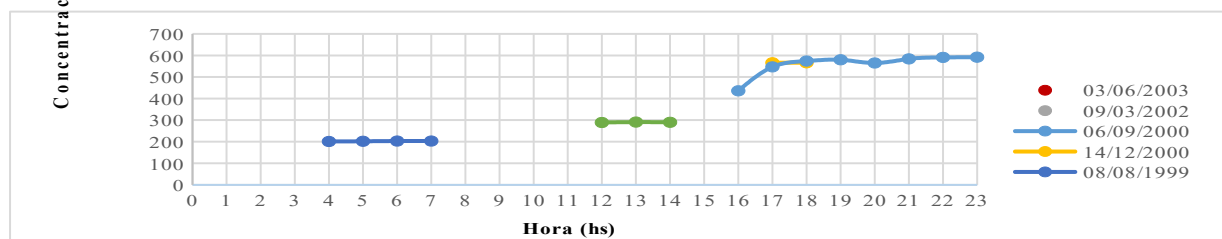
Figura 1. Concentración media horaria de SO 2 (ppb) en función del horario registrado para eventos sin vientos calmos.
