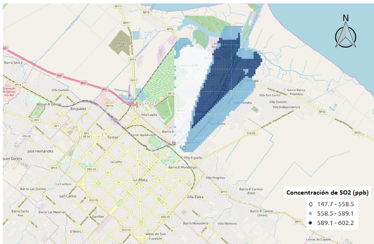
Figura 5. Aplicación del modelo NTA: Concentraciones promedio para el evento desarrollado el día 6-Septiembre-2000 entre las 16 y 23 horas. El círculo blanco marca la ubicación geográfica del sitio receptor.
