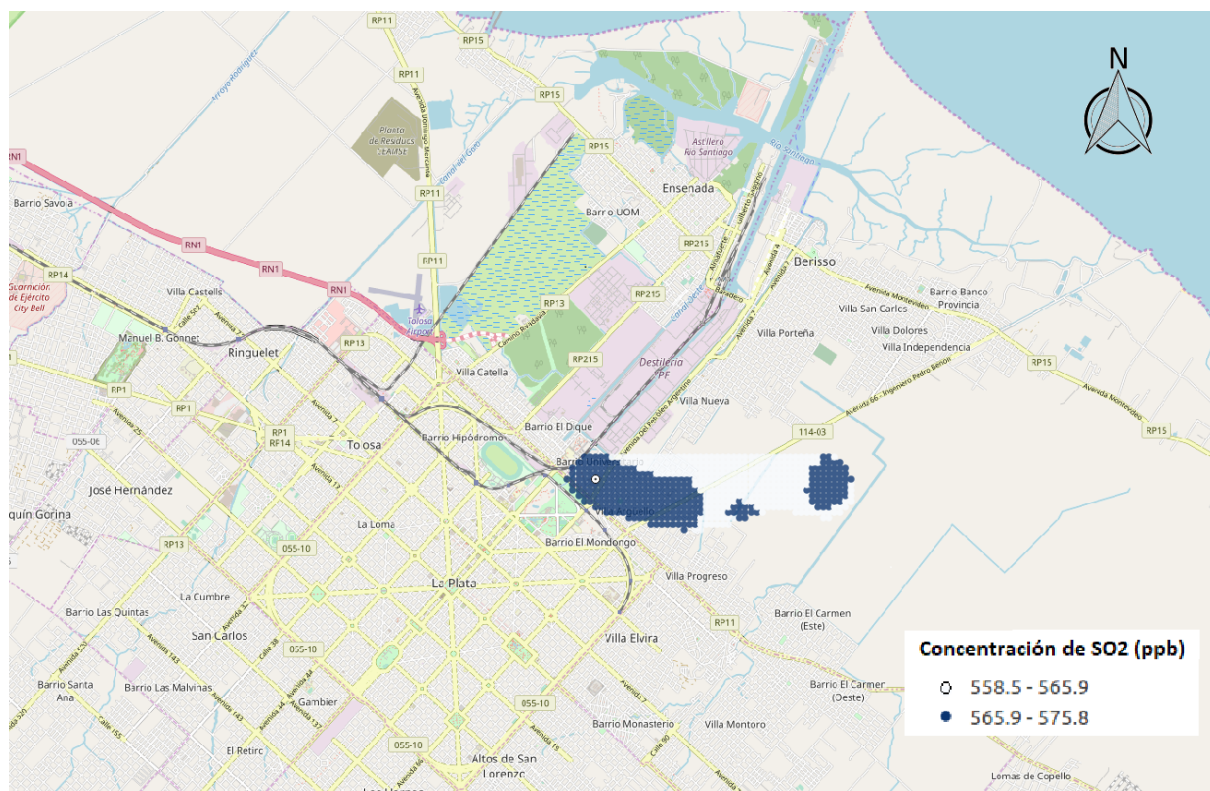
Figura 6. Aplicación del modelo NTA: Concentraciones promedio para el evento desarrollado el día 14-Diciembre-2000 entre las 16 y 17 horas. El círculo blanco marca la ubicación geográfica del sitio receptor.
