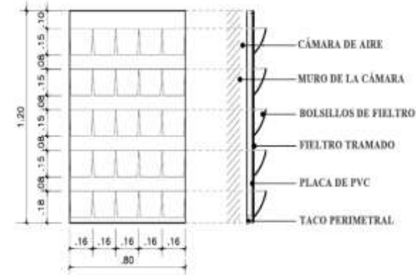
Figura 2. Esquema del módulo (frente y perfil).
