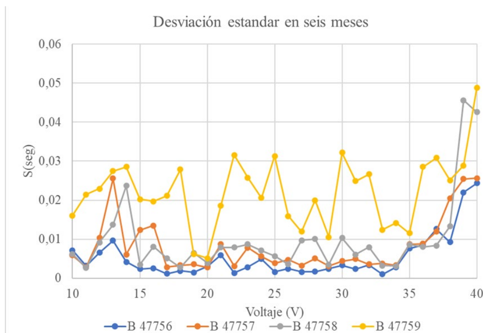
Figura 3. Desviación estándar de los seis meses de prueba de los datos obtenidos en el banco de pruebas.
