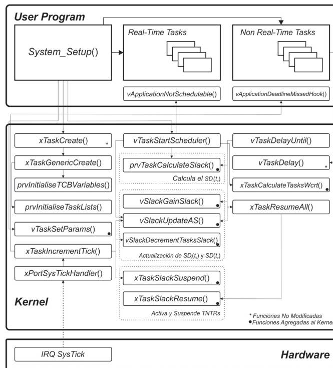
Fig. 2. Modificaciones y Agregados al Kernel del FreeRTOS.
